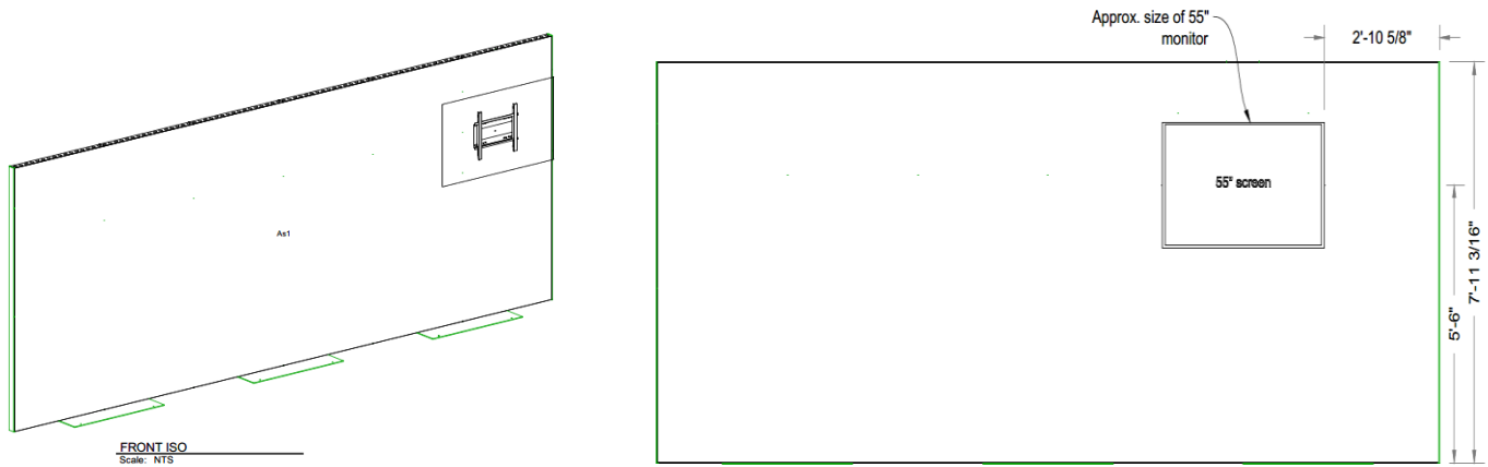
Backwall As1 Panel: 234.125"W x 95"H
