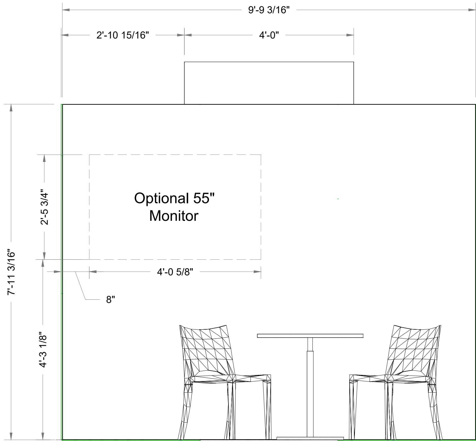
FRONT Scale: 3/4" = 1'
