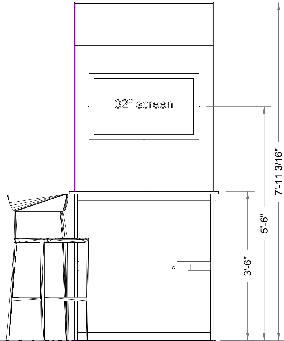
FRONT Scale: 3/4" = 1'
